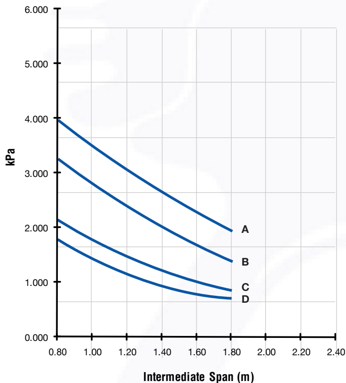
T - Rib 0.40mm UDL
