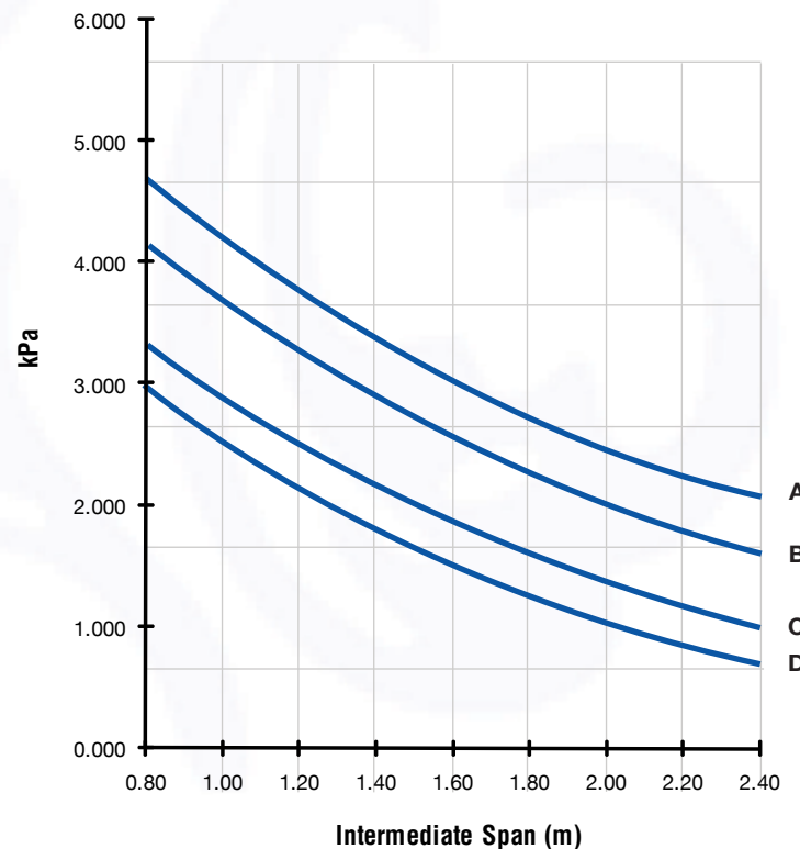
T - Rib 0.55mm UDL
